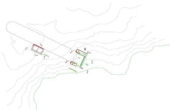
Figur 2 – Färjfastets vinkel
